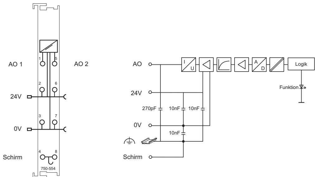
Abb. 2.1.1-3: 2-Kanal Analog Ausgangsklemme 750-554
