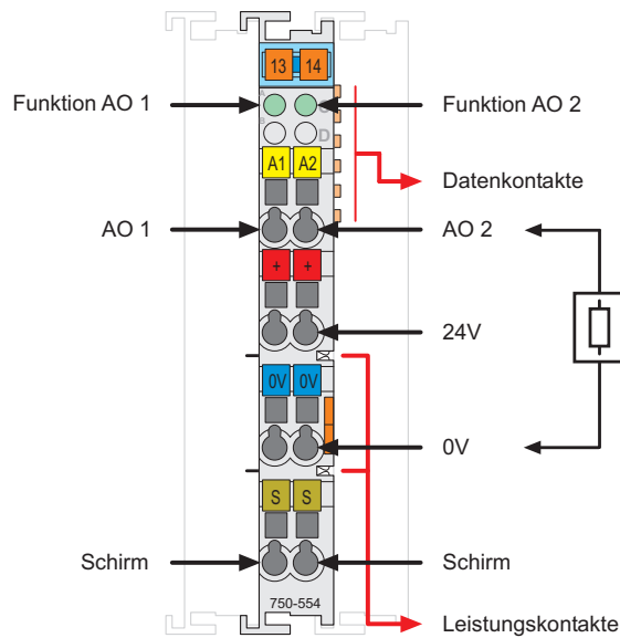
Abb. 2.1.1-1: 2-Kanal Analog Ausgangsklemme 750-554
